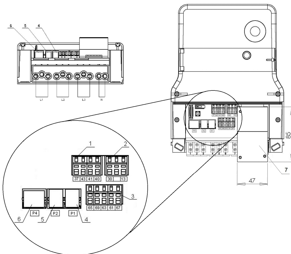
Izgled i dimenzije kućišta brojila kada se ne ugrađuje komunikacioni modem
