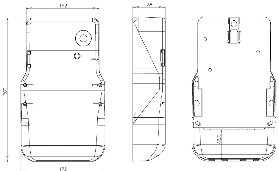
Izgled i dimenzije kućišta brojila kada se ne ugrađuje komunikacioni modem
