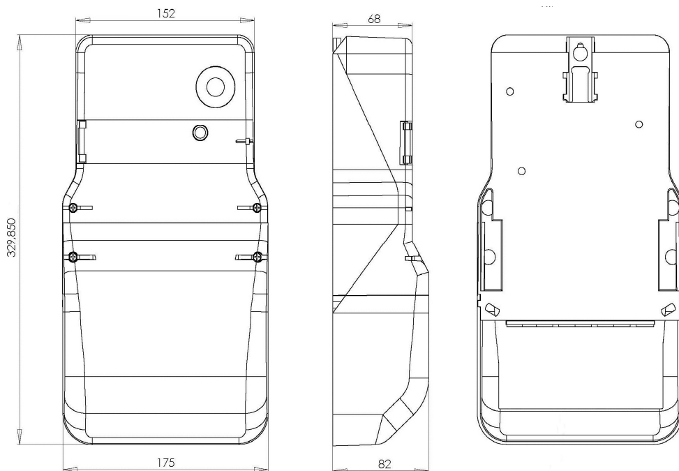
Izgled i dimenzije kućišta brojila kada se ugrađuje komunikacioni modem
