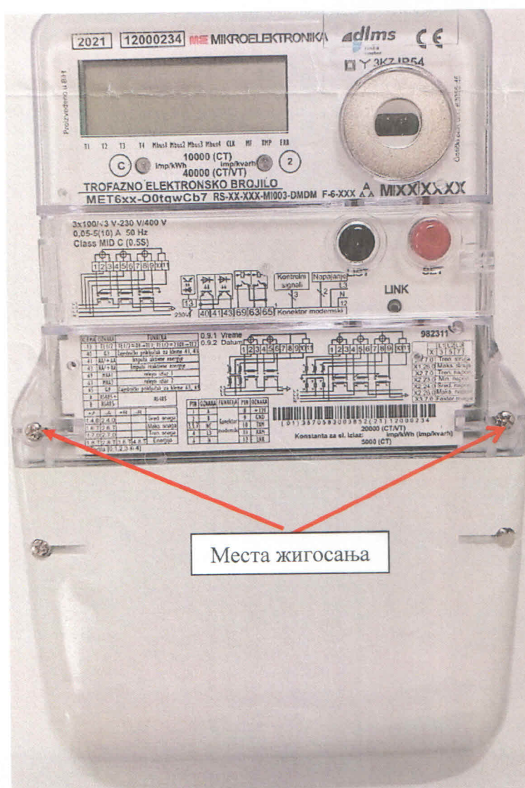
Слика 2. Изглед бројила и пример постављања жигова на пломбе
